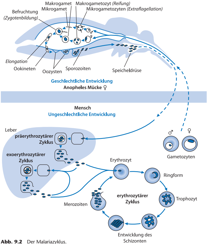
Abb. 9.2 Der Malariazyklus.
